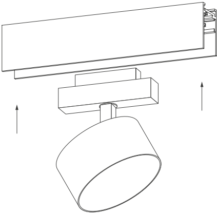
Рис. 2. Установка светильника
