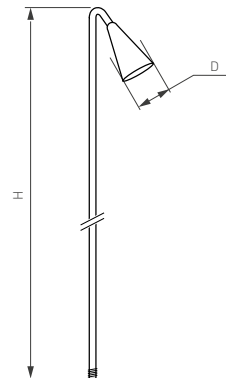
Рис. 1. Чертеж и габаритные размеры
