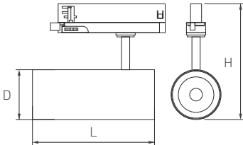
Рис. 1. Чертеж и габаритные размеры
